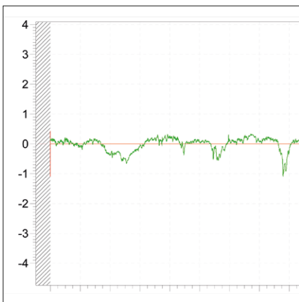
RENNSTEIG Splintentreiber Ra : 0,15 µm, Rz : 0,92 µm
