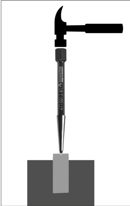
festsetzende Schraube mittig kören
