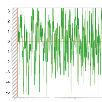
Splintentreiber Vergleichsprodukt Ra : 1,53 µm, Rz : 11,13 µm
